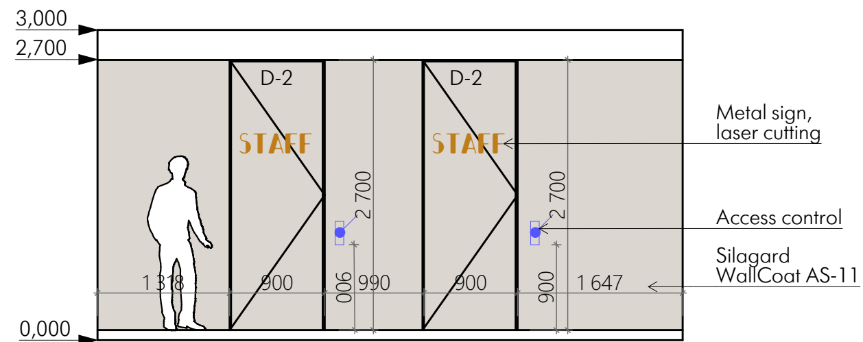
Wall L-M
